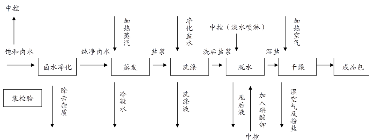
图 5-12 食用盐生产流程
