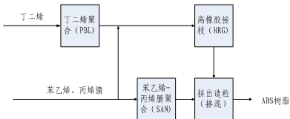
图 5-8 ABS 树脂制取流程示意图
