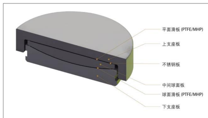
球型钢支座结构示意图：
