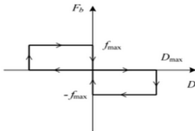
图1 BIO隔震系统中生物耗能元件的力学模型
