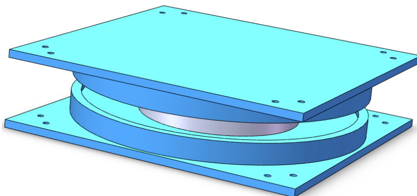
抗拉型摩擦复摆隔震支座（RB-FPB（L））：
