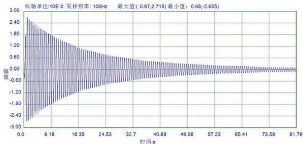
原结构加速度时程
