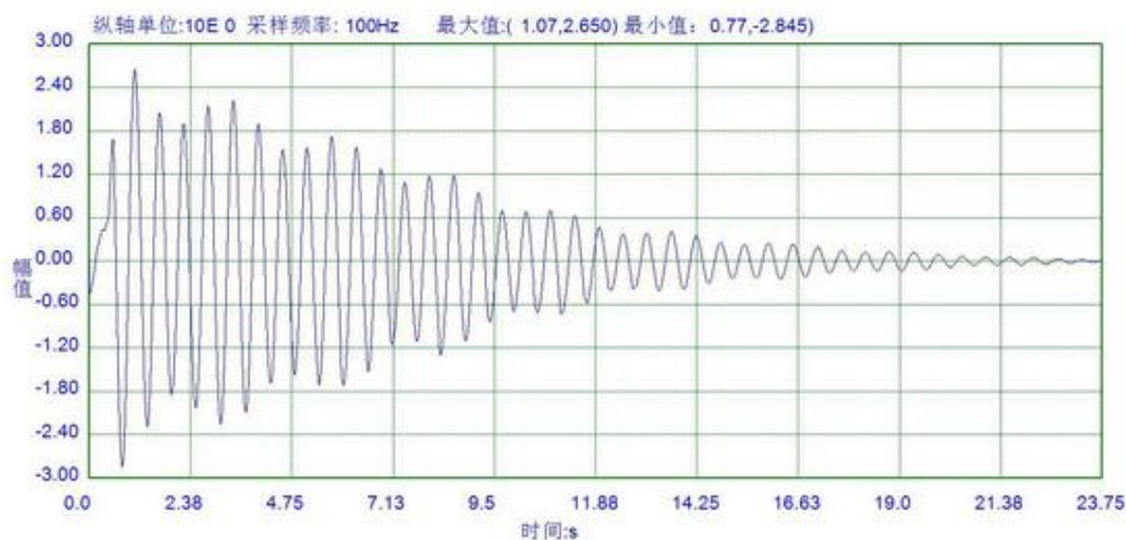
悬吊自适应单摆式TMD后的加速度时程曲线
