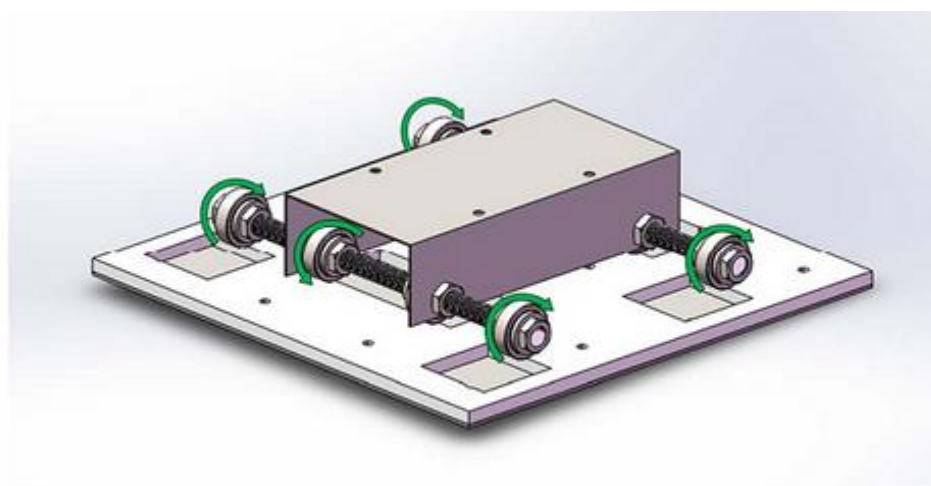
图2 BIO隔震装置示意图
